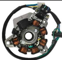
ESTATOR COMPLETO TITAN 99 /XLR
